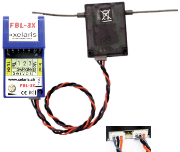
Anschluss der Spektrum Satelliten Empfänger
